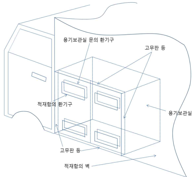
그림 2-1 용기보관실 문에 환기구 설치
