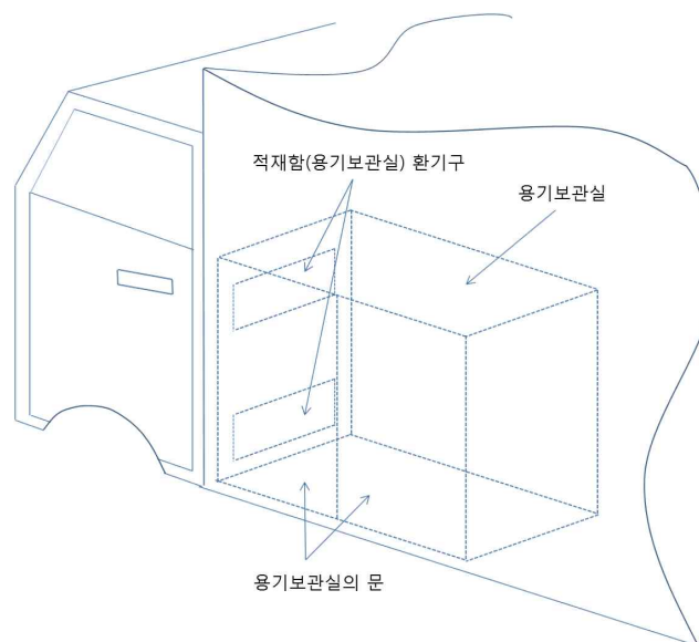
그림 2-2 적재함(용기보관실)에 환기구 설치
